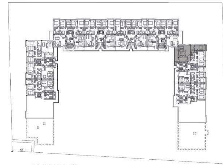
VIVIENDA 49 PLANTA SEGUNDA
